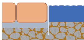
インターロッキングと アスファルトの見切
