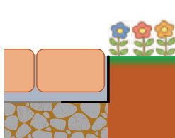
インターロックングと 緑地の見切 (ロックンエッジ・先施工)
