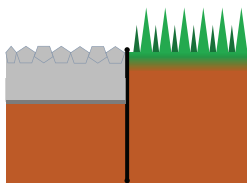
砂利と芝の見切
