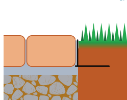
インターロックングと 緑地の見切 (ブリックエッジ)
